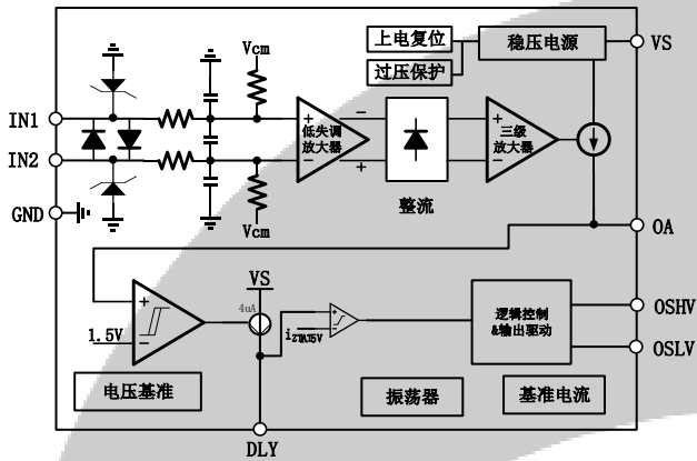
Figure 5. 芯片内部框图
