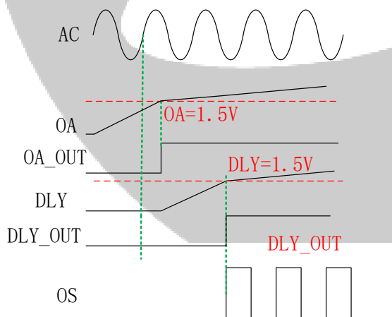
Figure 6. 工作原理图
