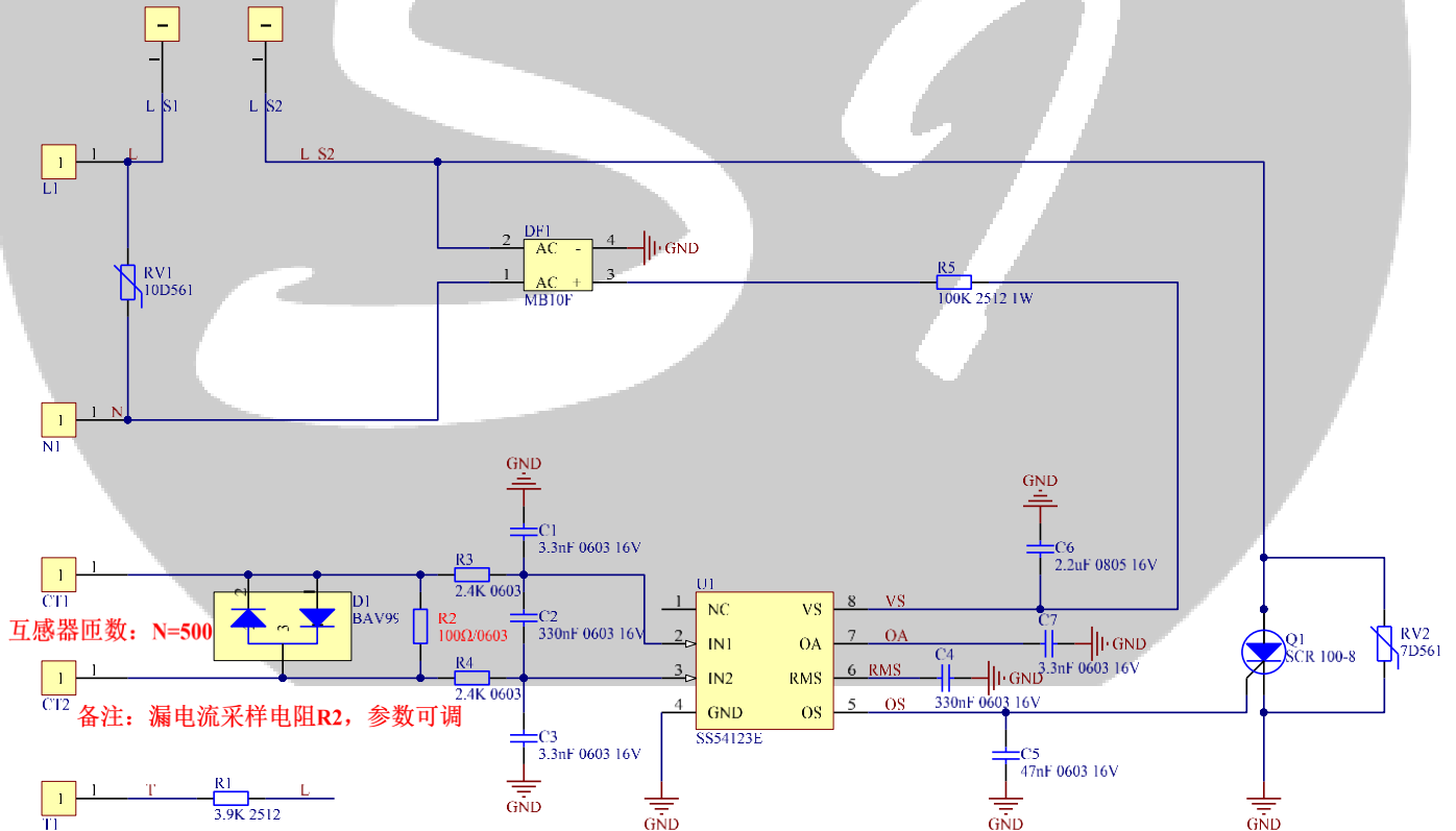
Figure 6. SS54123E 典型应用电路
